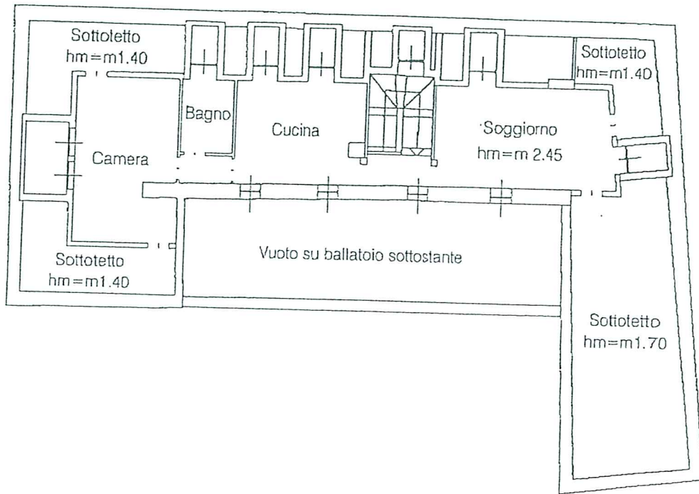
PIANTA PIANO SECONDO ( SOTTOTETTO )
